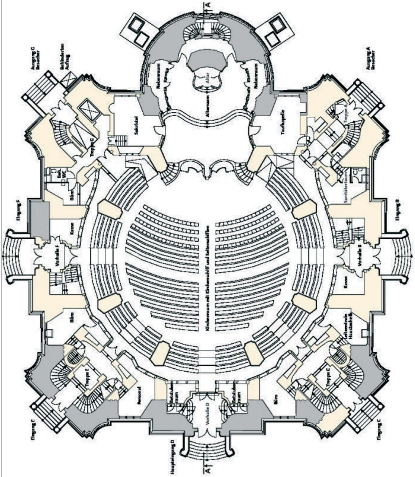
Grundriss Erdgeschoss, M 1 : 333 1/3
